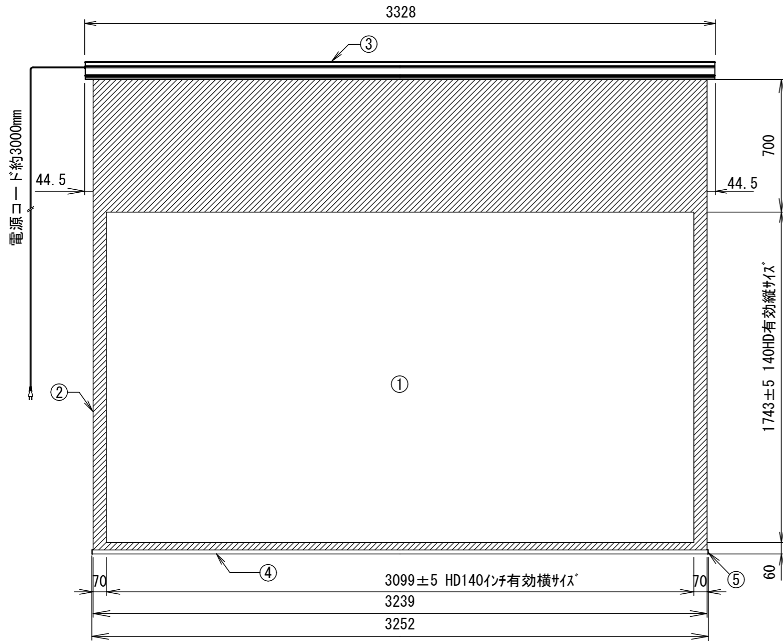
正面図
