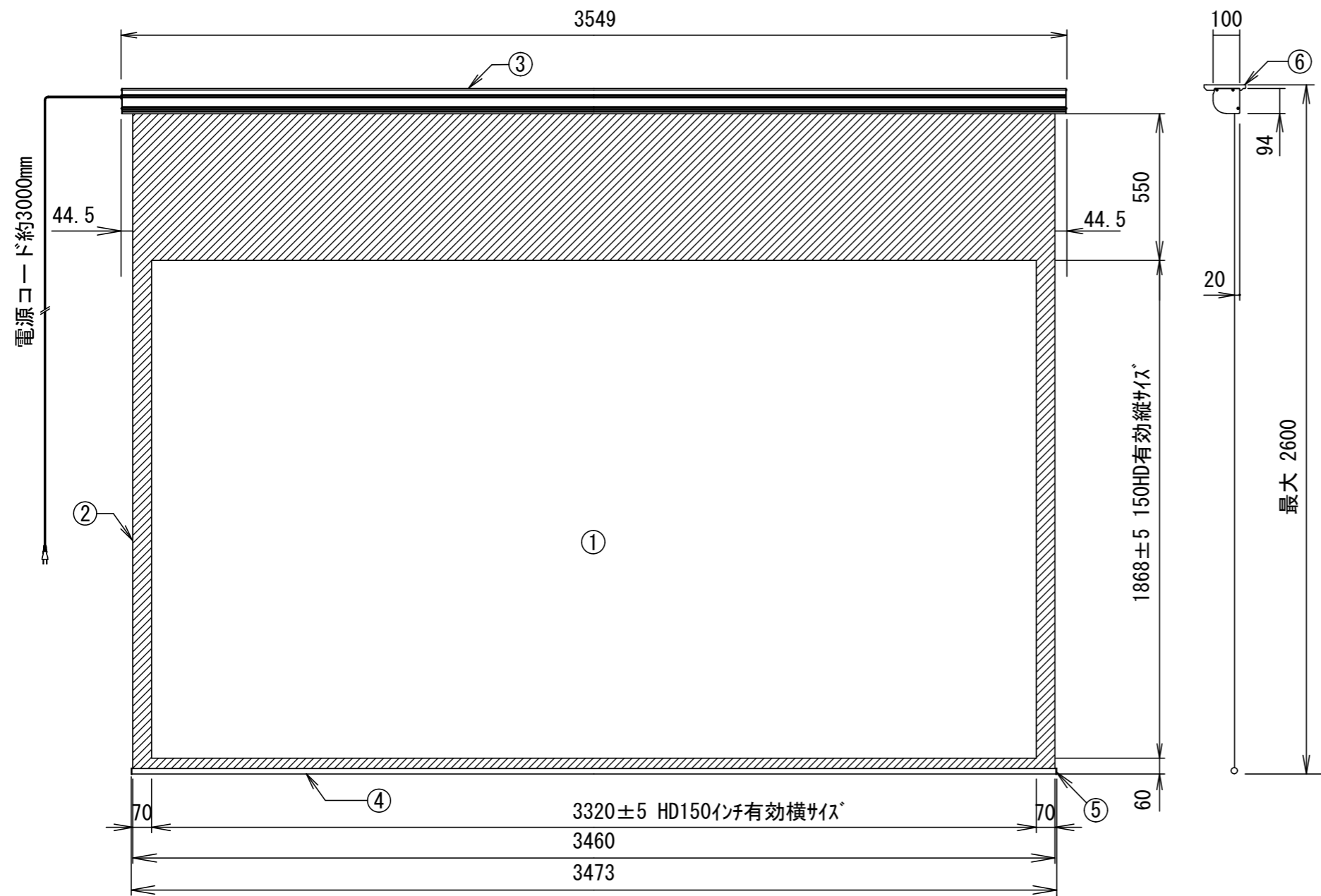
正面図
