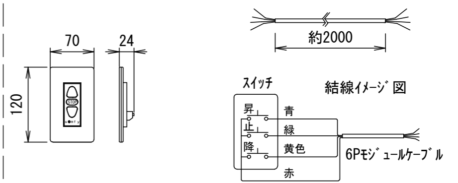
壁埋込非自照スイッチ (GSW-1)
