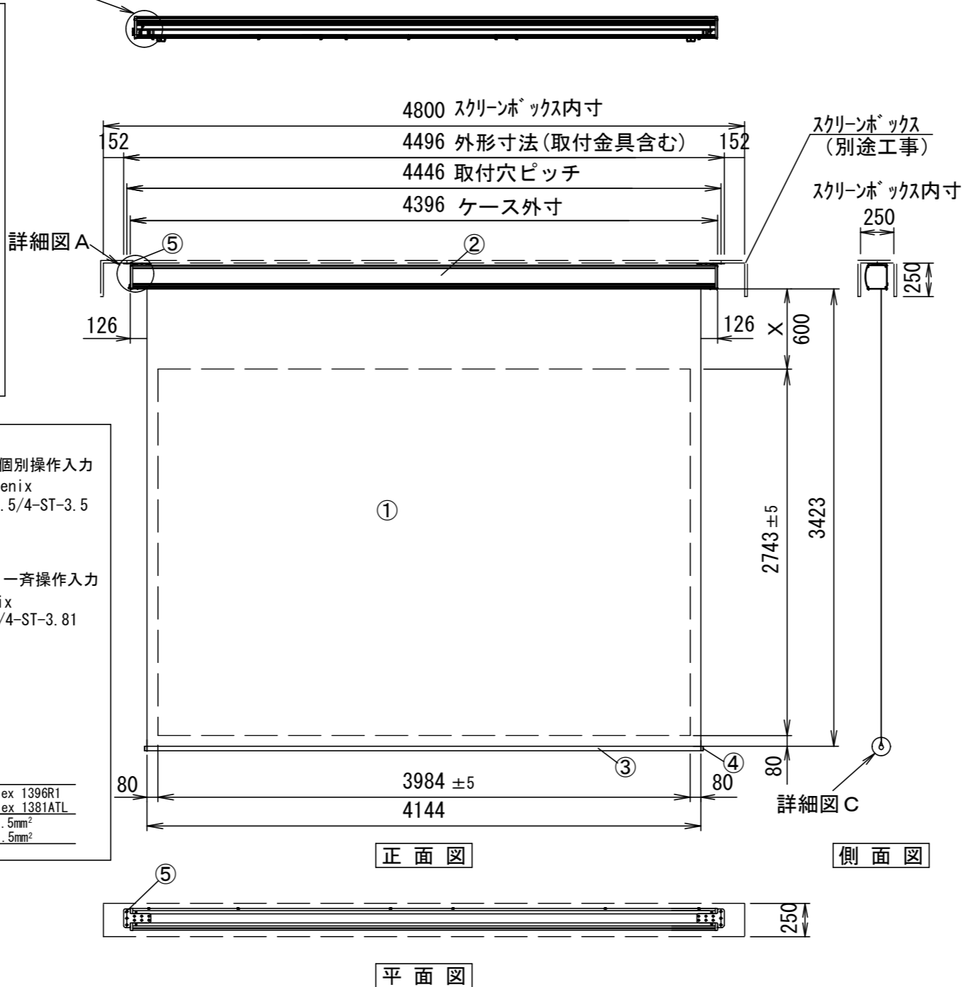
詳細図 B
