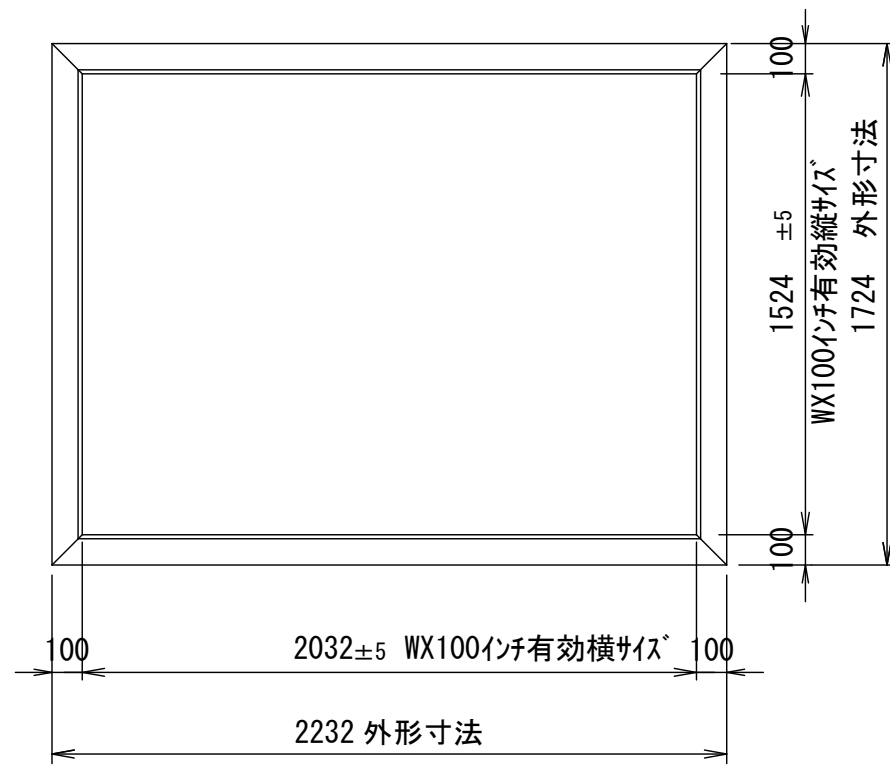
正面図
