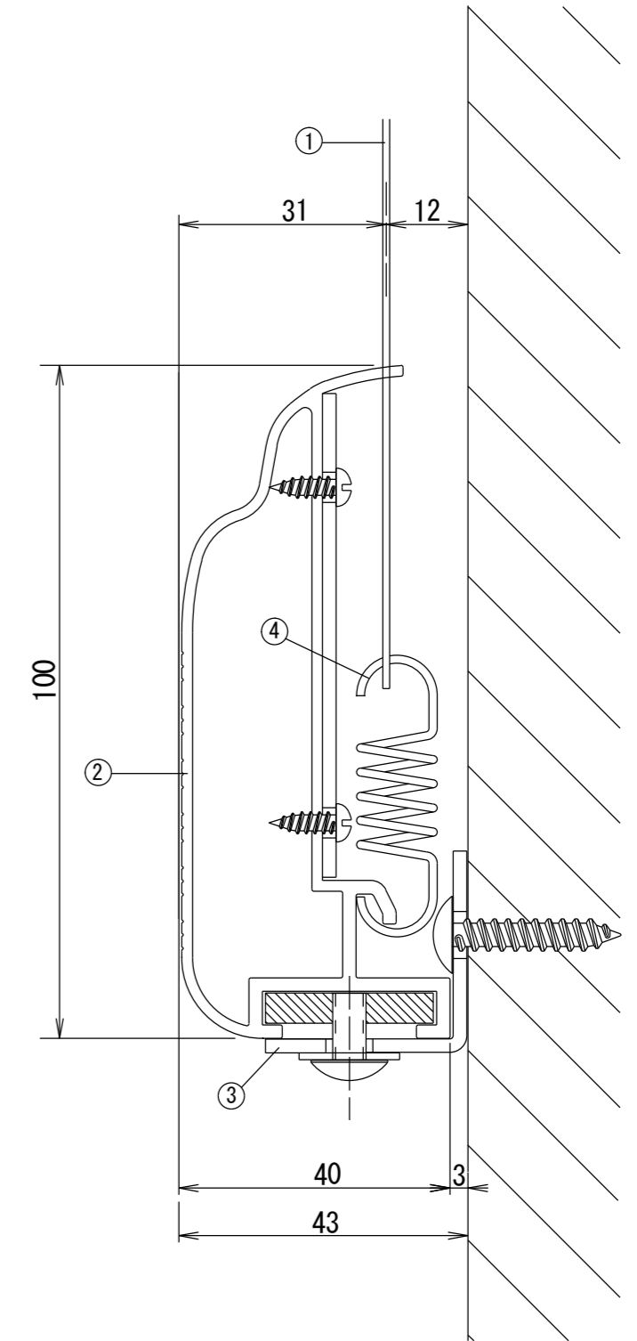
A 断面図 S = 1 / 1
