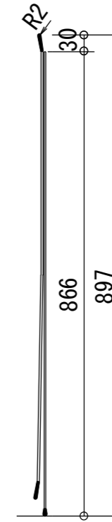
ワイヤースタンド
