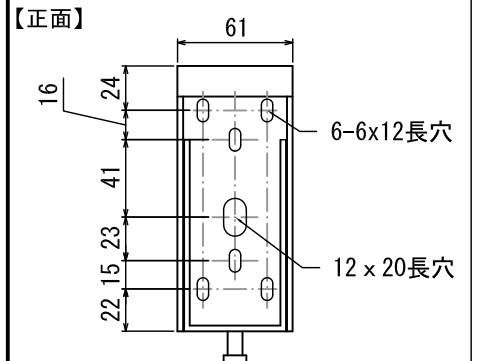
セッティングブラケット取付穴位置 S=1:4
