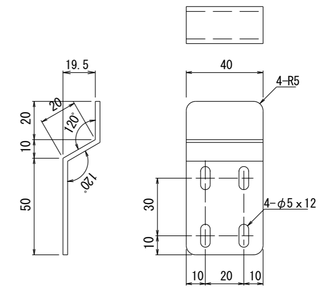
壁面取り付け金具寸法図
