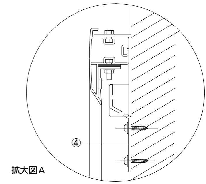
壁面取り付け状態
