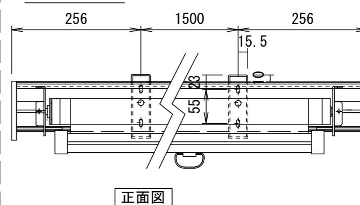
壁面取付時
