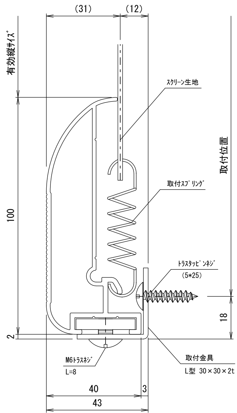
A断面図 S = 1 / 1
