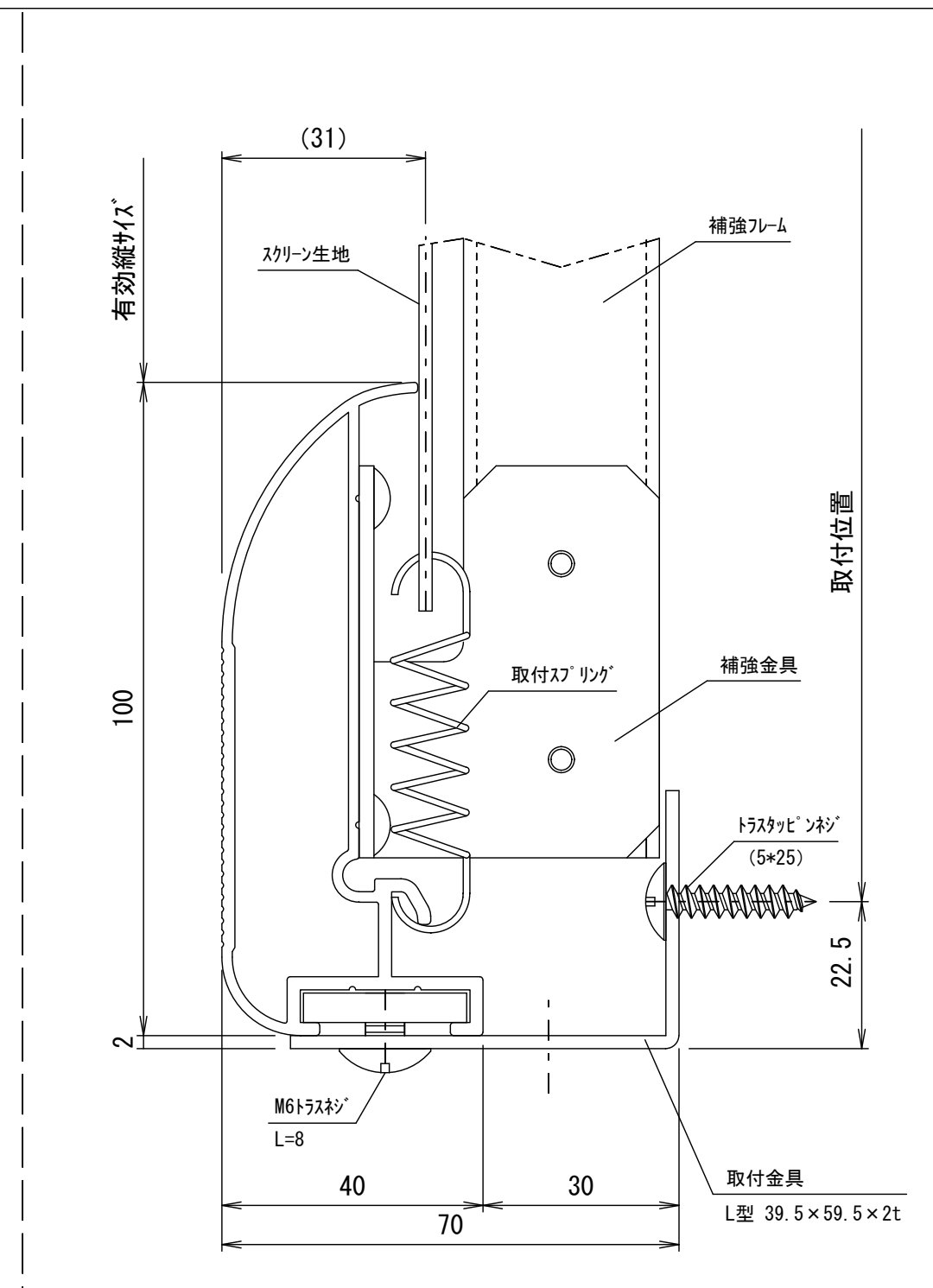
A 断面図 S = 1 / 1
