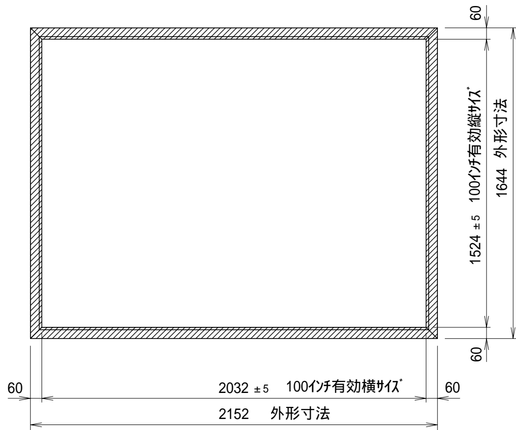
正面図
