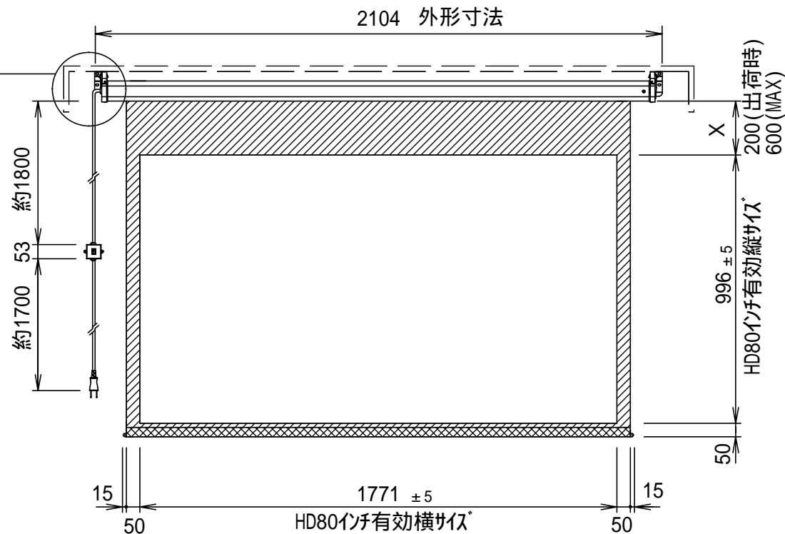
正面図
