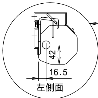
電源コード位置
