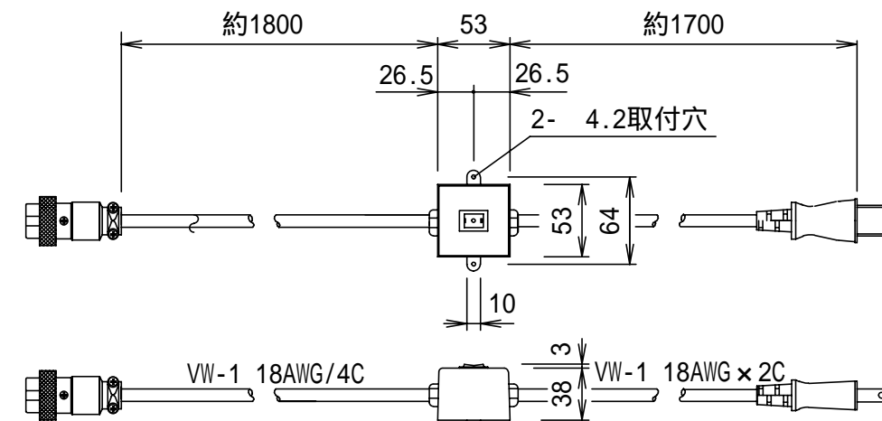
付属電源スイッチコード
