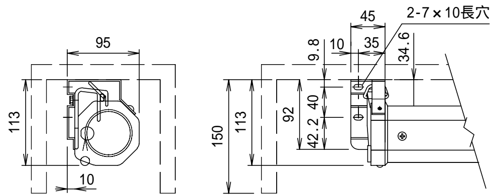
詳細図 SCALE = 1 / 5
