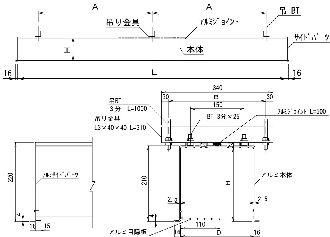
200型アルミボックス
