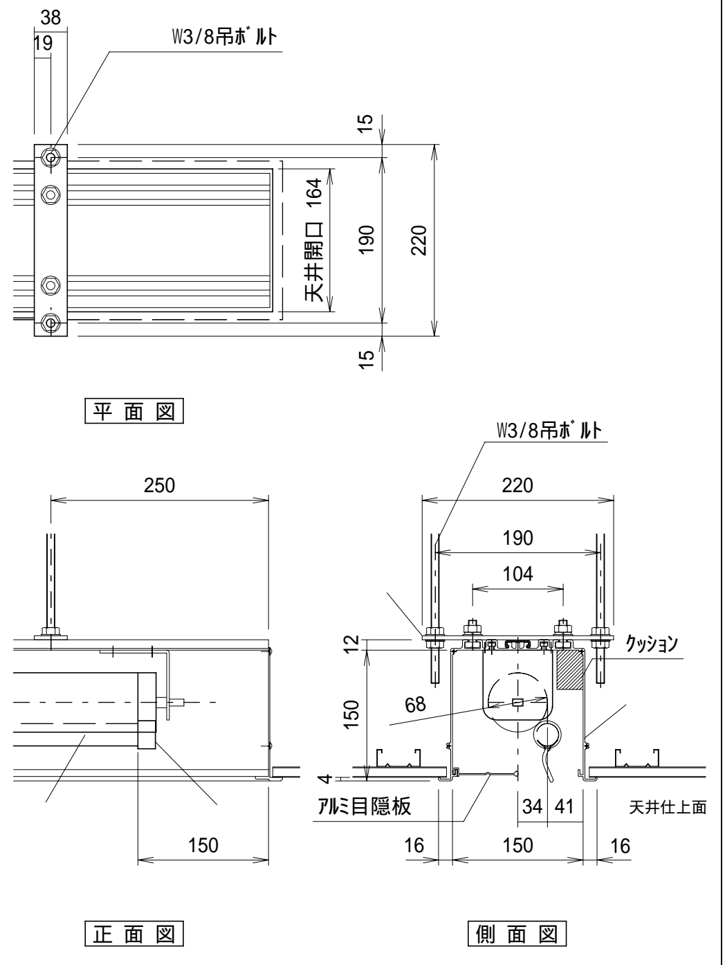
詳細図 S = 1/6
