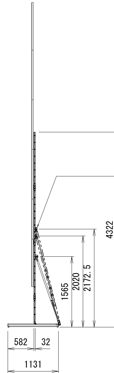
AT-32/64-Leg
