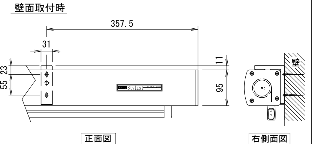
詳細図S=1/6
