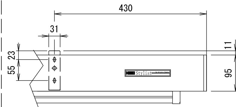
正面図
