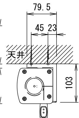
右側面図
