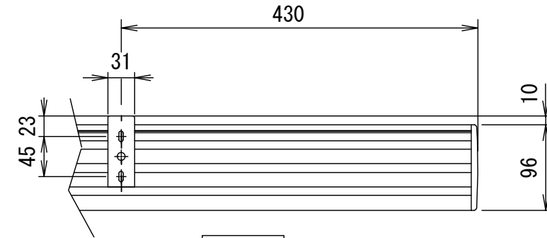
平面図
