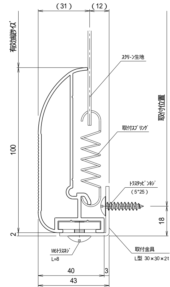
A 断面図 S = 1 / 1
