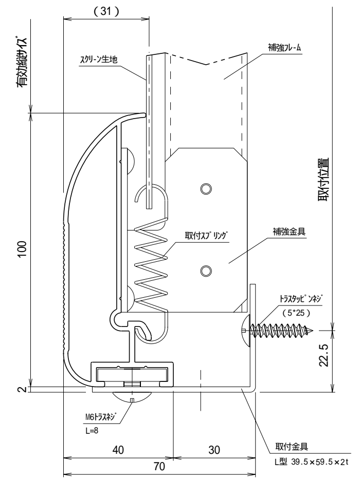
A 断面図 S = 1 / 1
