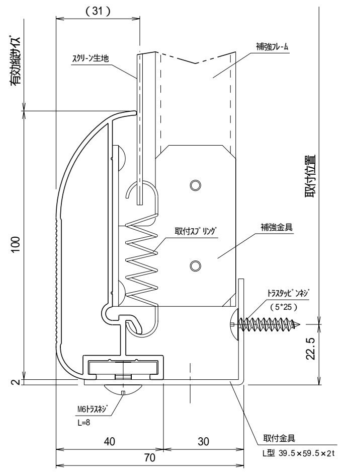
A 断面図 S = 1 / 1
