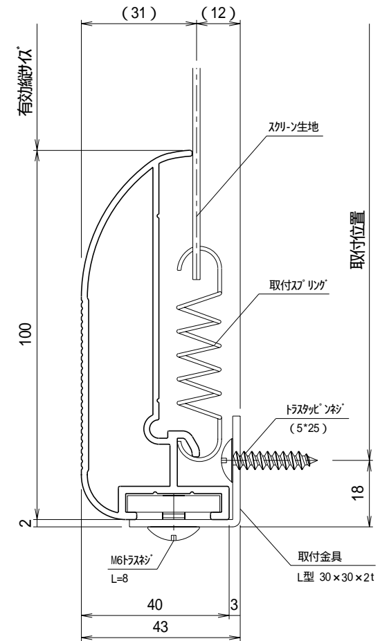
A 断面図 S = 1 / 1
