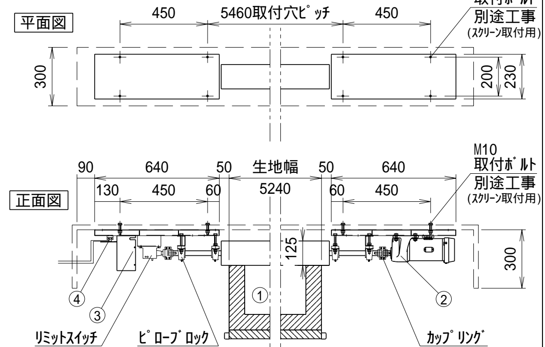
詳細図S=1/20
