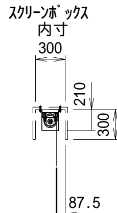
詳細図S=1/20
