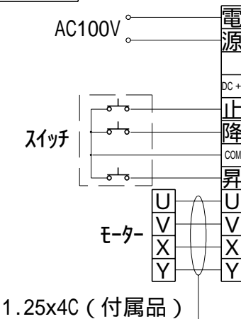
結線図
