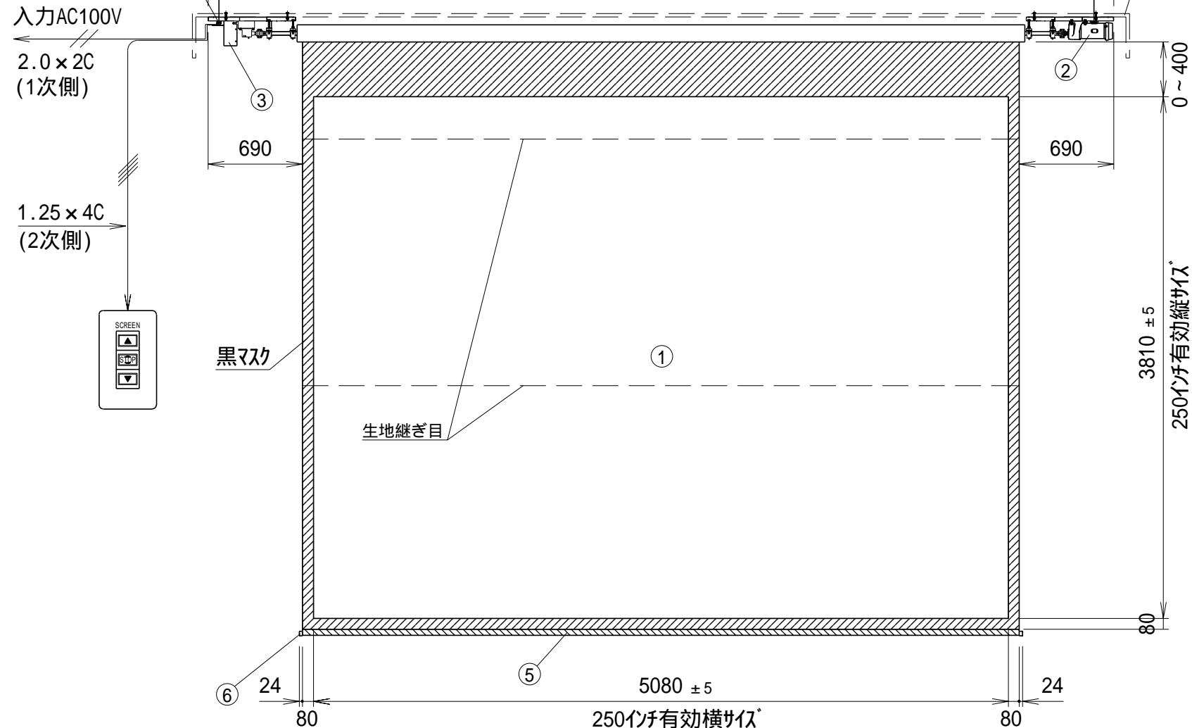
正面図
