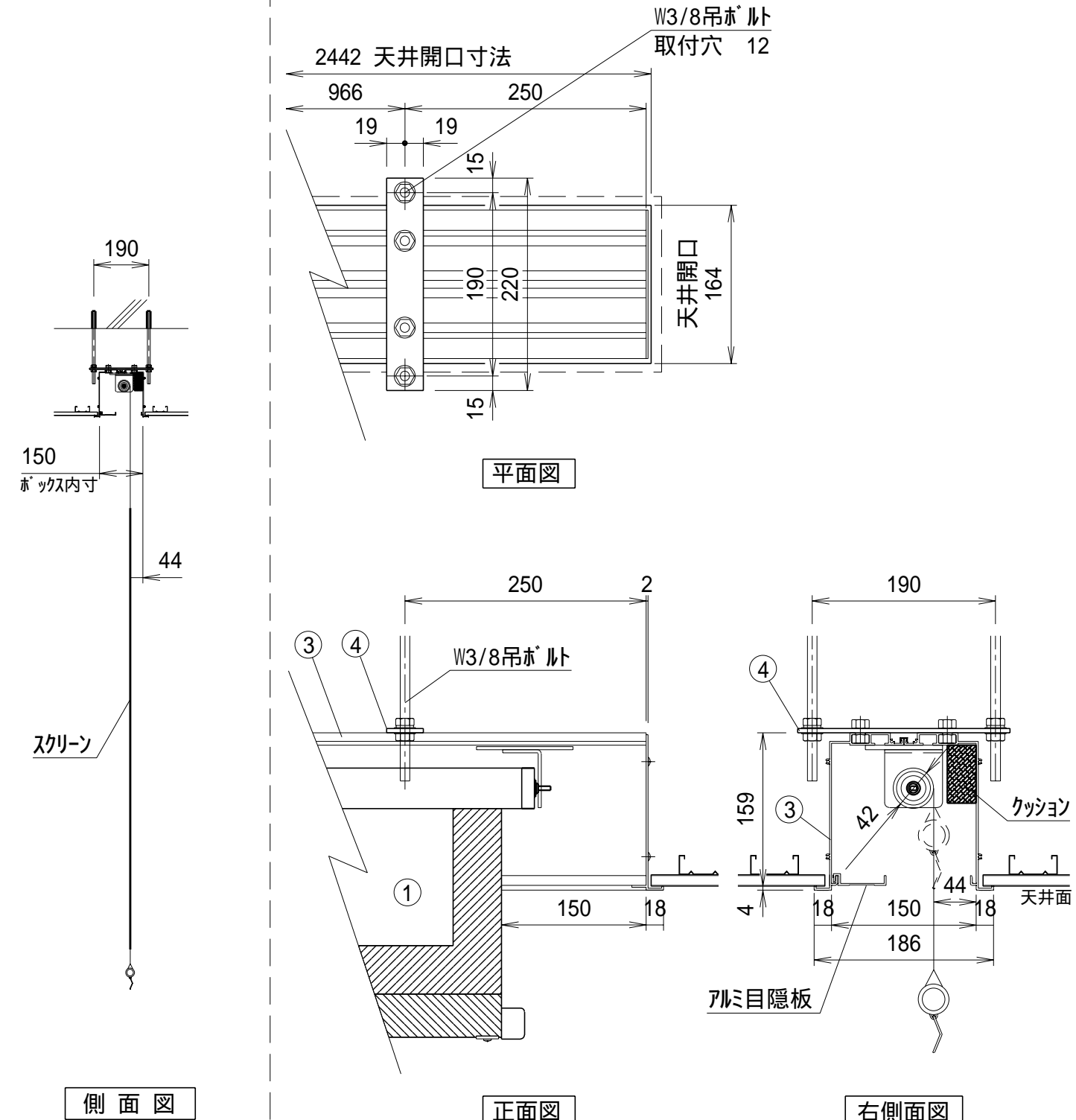
詳細図S=1/6
