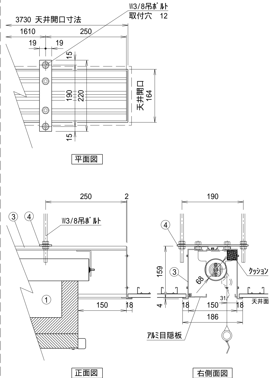
詳細図S=1/6
