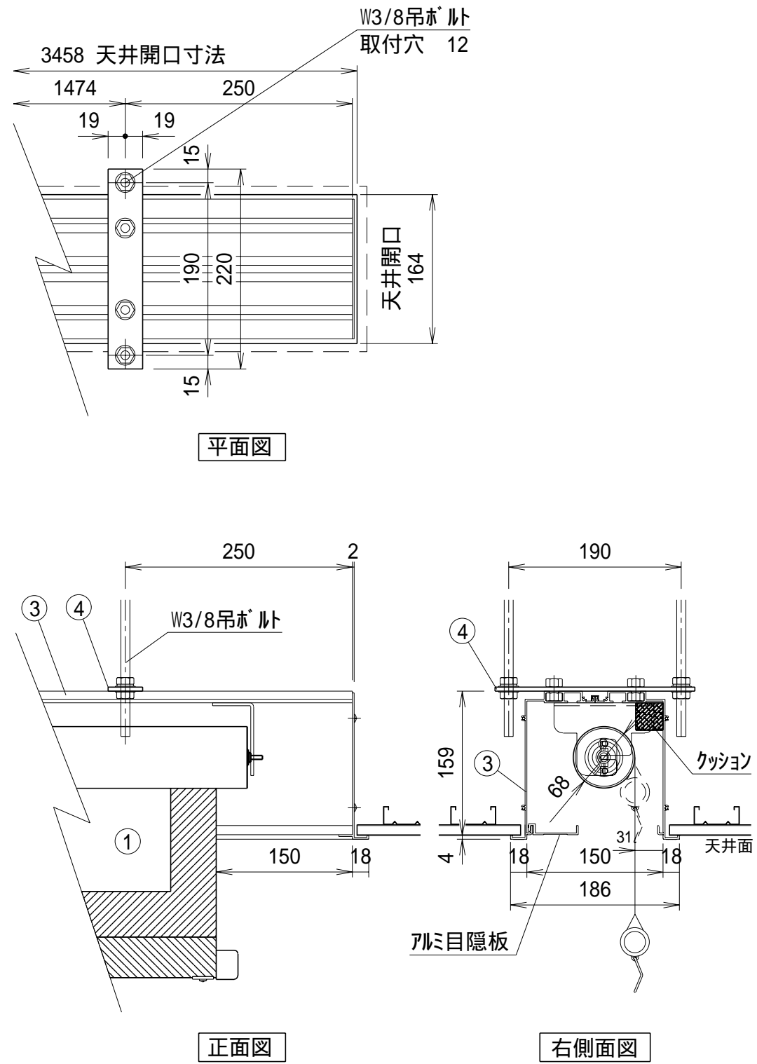
詳細図S=1/6
