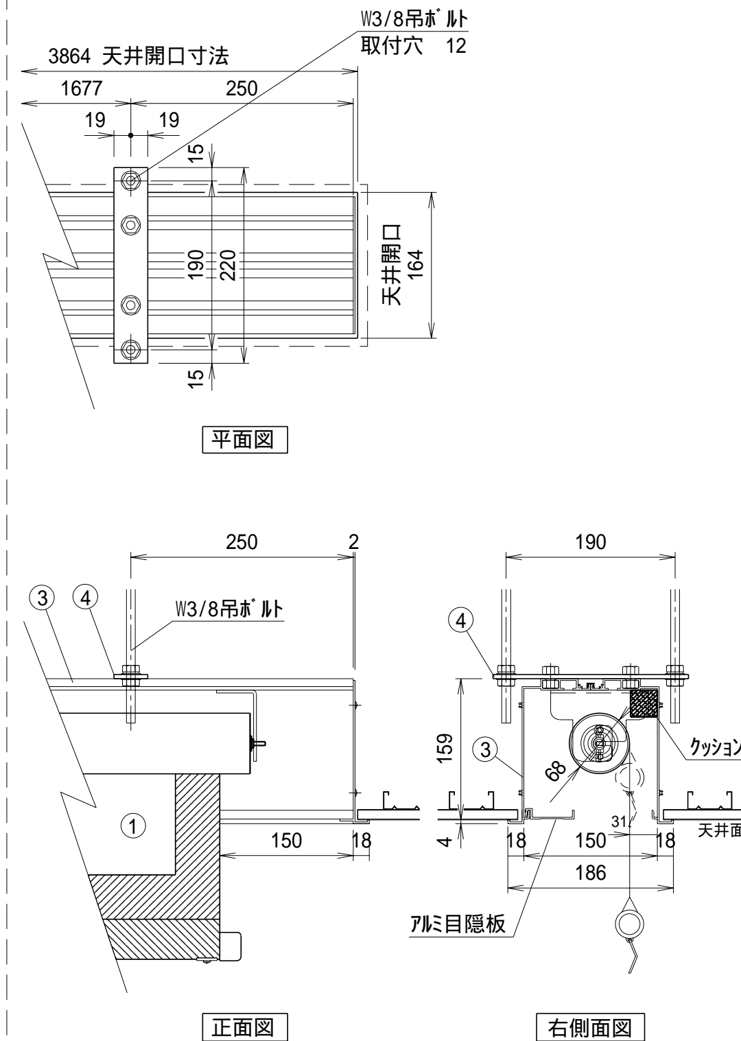
詳細図S=1/6
