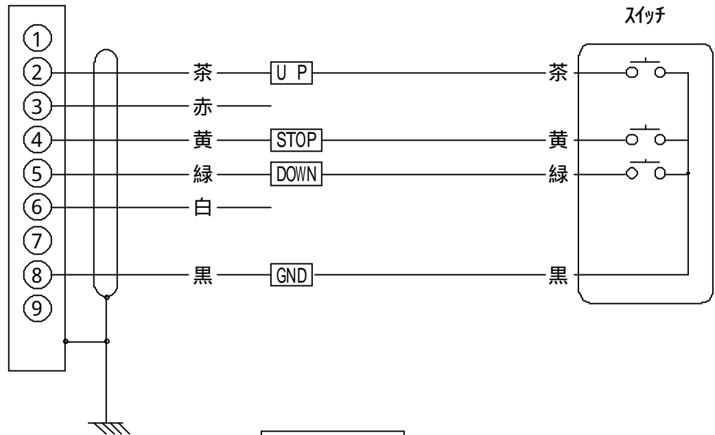
回路図
