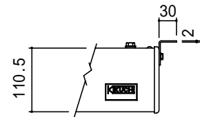
ケース 右正面図
