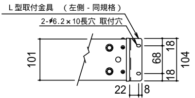
ケース 右平面図
