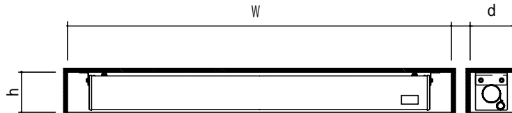
天井埋込ボックス 参考寸法(内寸法)
