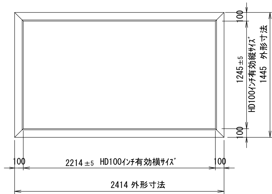
正面図
