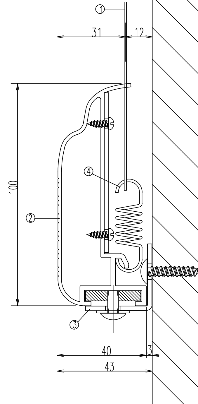
A 断面図 S = 1 / 1
