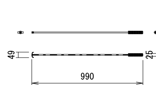
プルバー (引下げ棒) S=1/20
