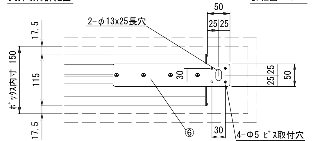
天井取付詳細図
