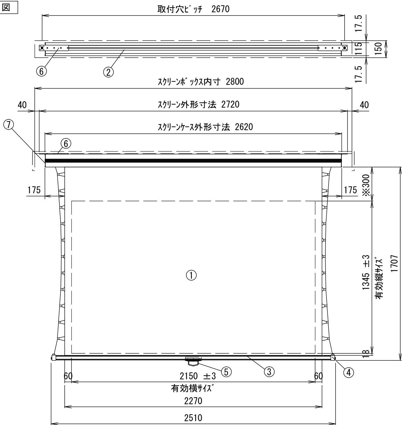
正面図
